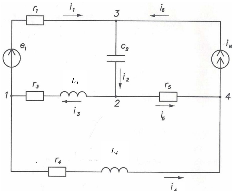
Рис. 1. Разветвленная электрическая цепь
