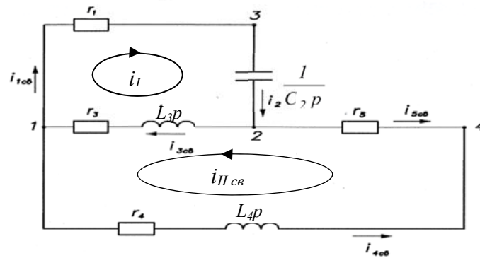
Рис. 2. Расчетная схема для определения свободных составляющих
